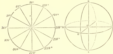
Fig. 1.—Plane Angles.
